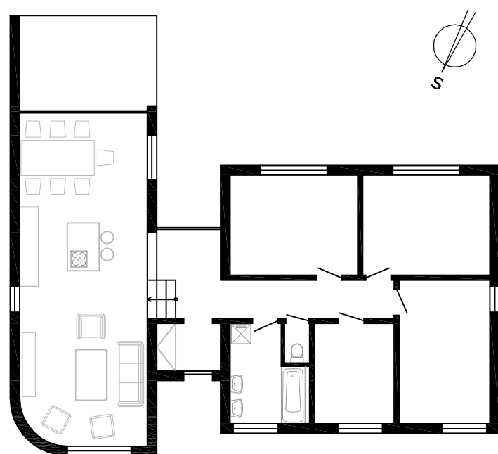
Půdorys 1.NP
